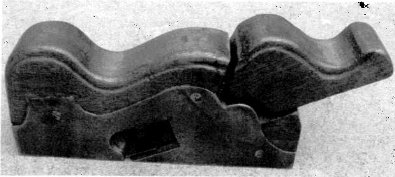
◀ Stalen boorschaaaf met mahonie inleg en spie. Engeland. Beitel 38 mm, geen merk.
