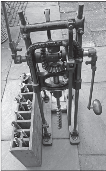
28. Mooie Millers Falls stoeltjesboor geheel compleet. Heel uniek hierbij is een kist waarin 12 originele boorzijzers zitten.
