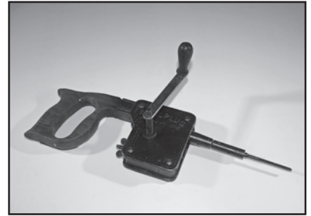
17. Rawlplug klopboormachine.
