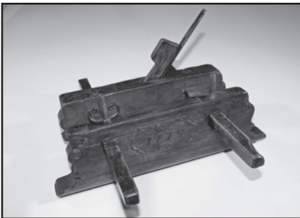
6. Hollandse veerploeg met datering 1774. Eén vleugelmoer ontbreekt. De Duesing beitel is niet origineel. Geen schavenmakersmerk.
