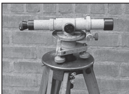
25. Waterpasinstrument op statief. Merk Ahrend. Type 6503.
