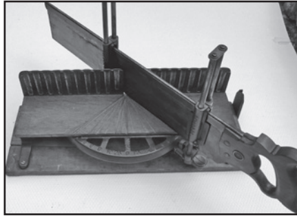
4. Prachtige complete verstekbak. De Disston ets op het zaakblad is goed bewaard.
